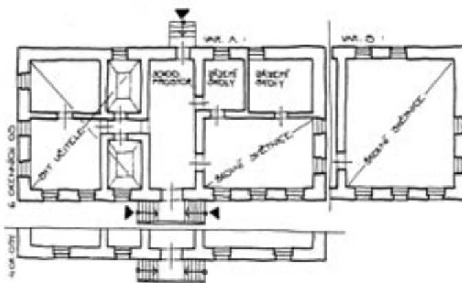
Obr. č. 1: Dispozice objektu staré školy při výstavbě z roku 1805. Kresba E.Kösslerová
