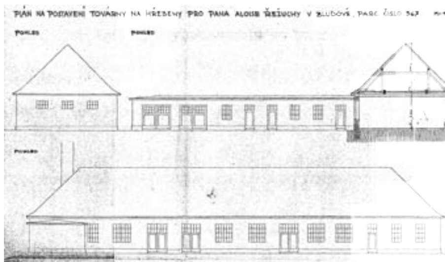
Plán na postavení továrny na hřebeny – výroba ve tvaru písmene L
